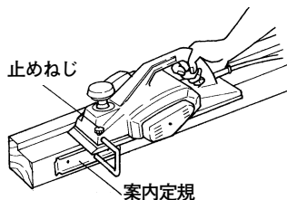
相じゃくり時の案内定規の取付け図
