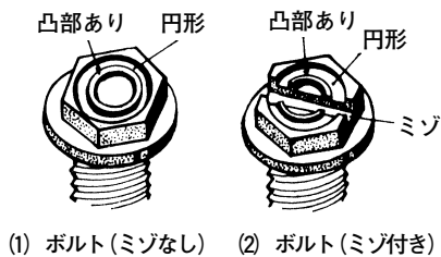
交換用ボルト頭の形状
